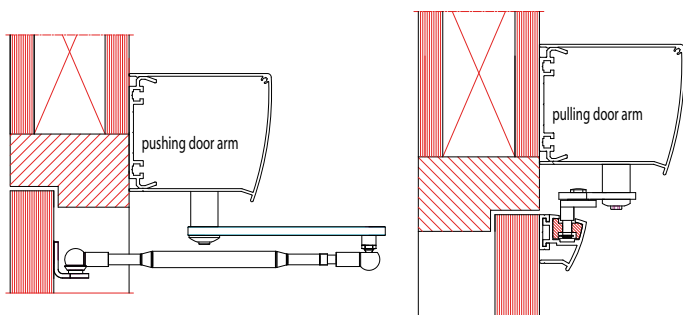
▲ Tvärsnitt över KONEs automatiska slagdörrar. ▲
