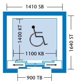
Behindertengerecht: 8 Personen/630 kg
