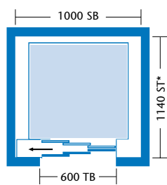
KONE ReNova Slim L4/C4 dreiteilige seitlich öffnende Tür
