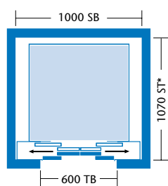
KONE ReNova Slim L3/C3 vierteilige zentral öffnende Tür
