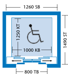
Behindertenfreundlich: 6 Personen/480 kg
