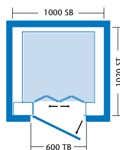
Drehtür mit vierteiliger Kabinen-Faltdür
